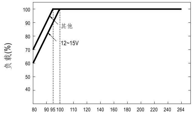
输入电压(VAC) 60Hz
